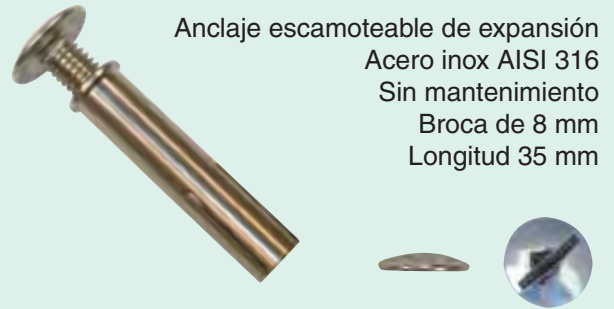
Anclaje de expansión acero inox AISI 316 Cabezal de inox revestido de nylon Sin mantenimiento Broca de 8 mm
